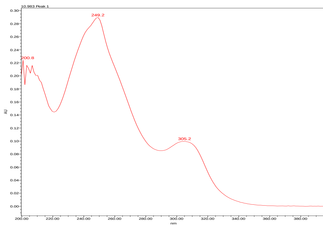
圖十三、葛根素的 UV 圖譜
