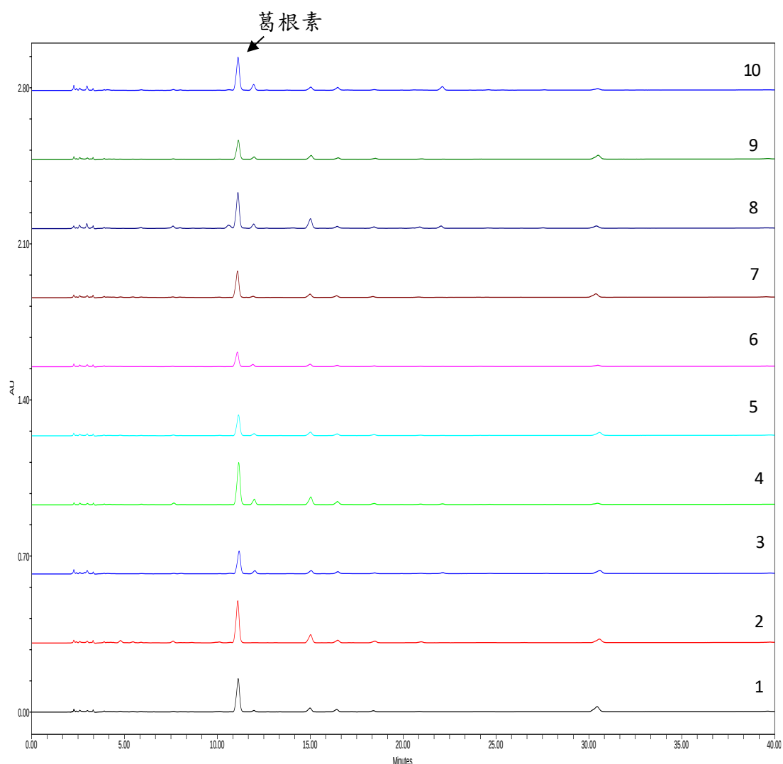
圖六、10 批粉葛藥材之 HPLC 層析圖
